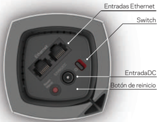
Parte inferior
