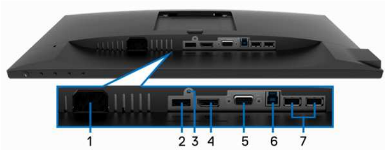
Vista inferior sin soporte de monitor
